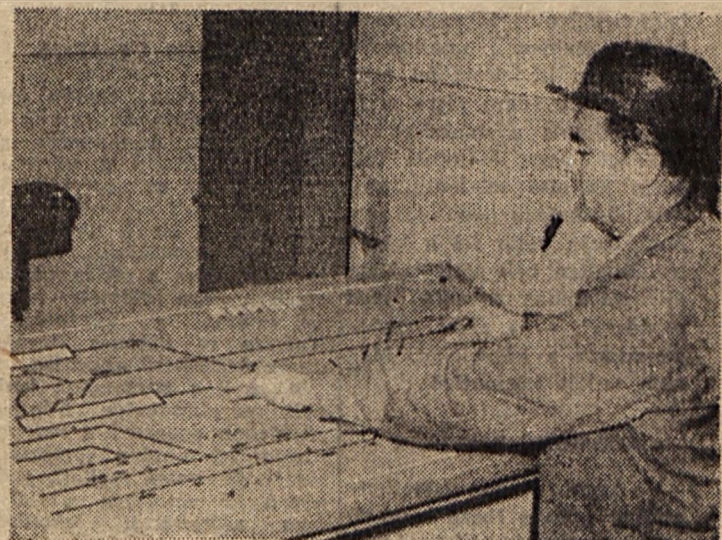
A Kossuth-bányai altáróban a legmodernebb „integrált” vasútbiztosító berendezéssel irányítják a forgalmat. Képünkön a vezérlőasztal és kezelője Preizer Ferenc diszpécser.
