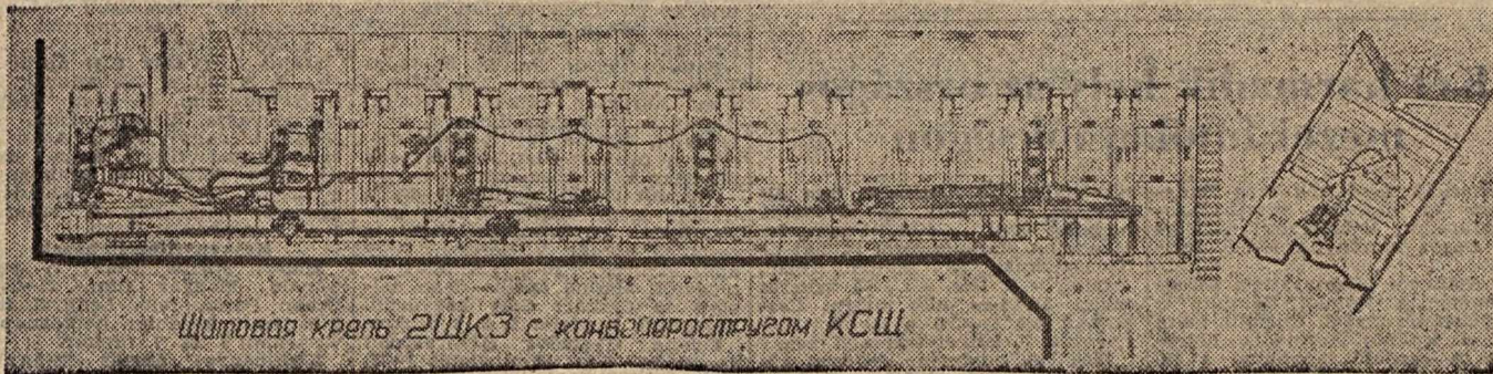
1. sz. ábra: Lépegető pajzs
