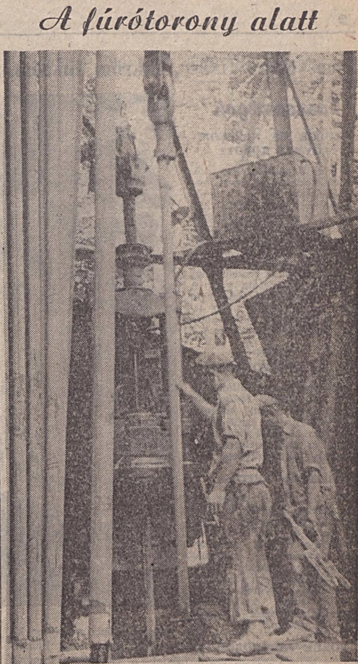
Munkában a mecseki szénvagyon kutatói. A Mecseki Földtani Kutató-Fúró Vállalat dolgozói nagy erőfeszítéseket tesznek első féléves lemaradásuk pótlására. Felvételünk a komlói Anna-akna melletti fúrásnál készült, Linder György fúrómester kollektívájának munkahelyén. (Foto: Berkics)
