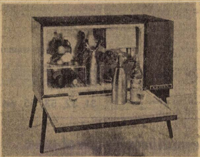
A Lehel szobahűtőszekrény tv-lábakra szerelve.
