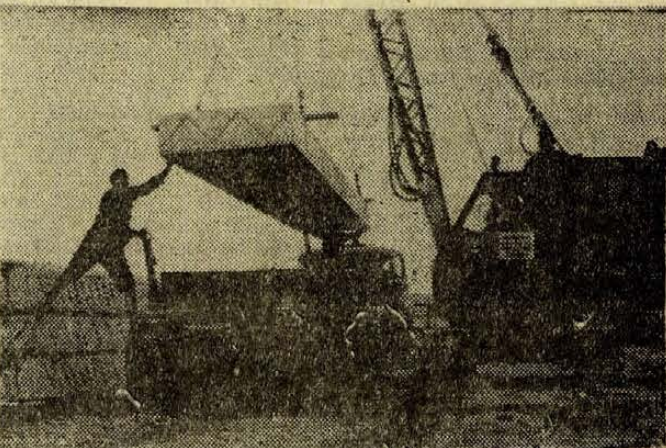
Íme az új, speciális építőanyag, a 3 és fél tonna súlyú, 12 méter hosszú, Semsey-panel. A szállításra egy 22 tonnás speciális vontatót alakítottak át és kétkerekű utánfutót készítettek hozzá.
