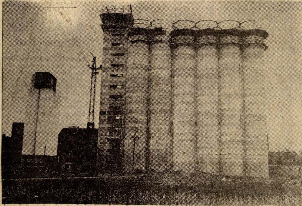
Egy hónap alatt fejezték be a hétszáz vagonos gabonátároló siló betonozását Pécsen a Fejlesztési útja mellett. Az építők három műszakban, éjjel-nappal dolgoztak. A silókat csúszsaluzással építették. Jelenleg a silók földmunkái folynak. Tervek szerint a 15 millió forintos beruházás átadásának végső határideje 1967. október 31. A gabonátároló teljesen gépesített lesz, közúti és vasúti hídmérleggel. (Foto: Szokolai)
