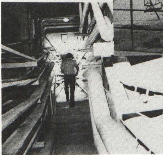
Közmű alagút a Lvov kertvárosban Pécs /1975/
