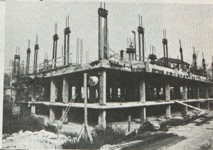
Megyei kórház földemének emelése/1974/
