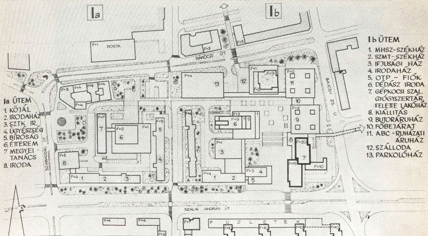
Városközpont beépítése. Pécs/1962/ Beépítési terv: Gerő Balázs, Köves Emil, Tilla Ernő Ybl díjasok.
