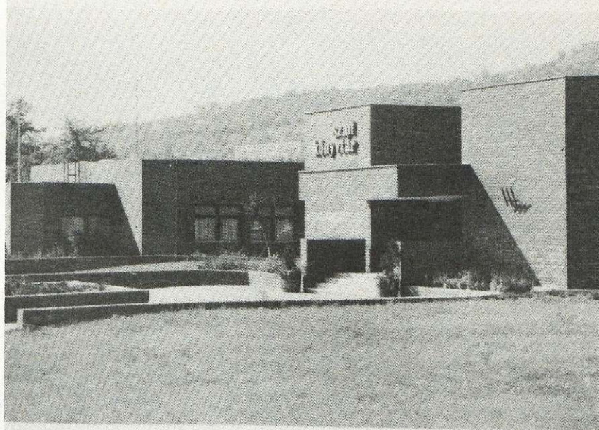
SZMT könyvtára. Pécs, Tüzér u./1981/ Építész: Várnagy Péter
