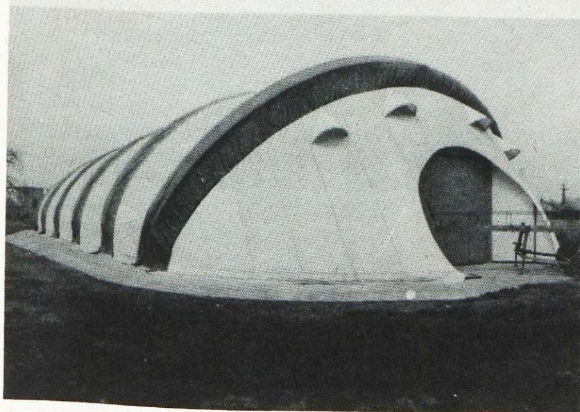
Sátor raktárak. Szekszárd és Dombóvár/1981/ Tervező: Dulánszky Jenő
