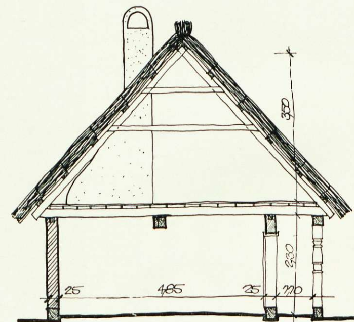
METSZET
