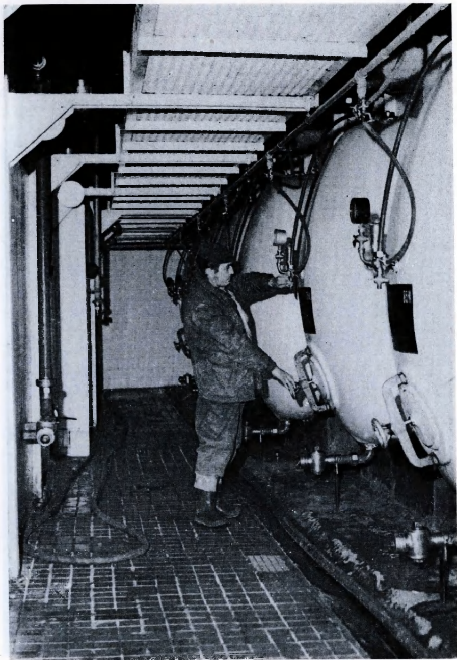
A falak mögött 60 óriási alumíniumtánc
