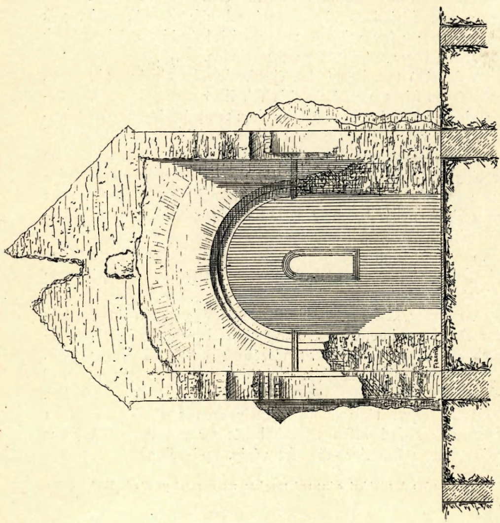
2. ábra. A széplaki templom szentélyének keresztmetszete.
