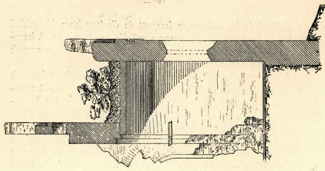
3. ábra. A széplaki templom szentélyének hosszmetsszete.
