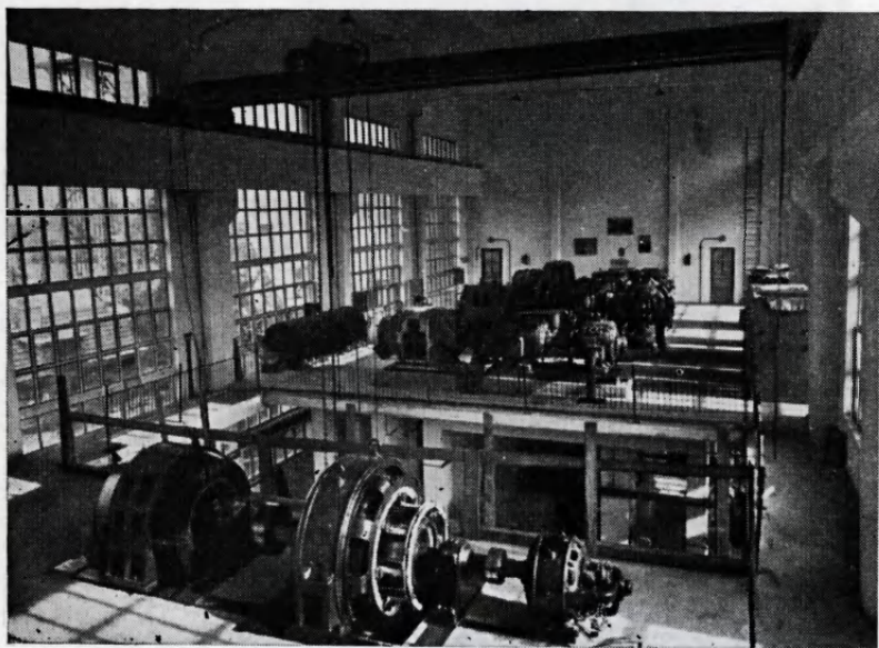
9. Gépterem a Kossuth-aknai kompresszorüzemben
