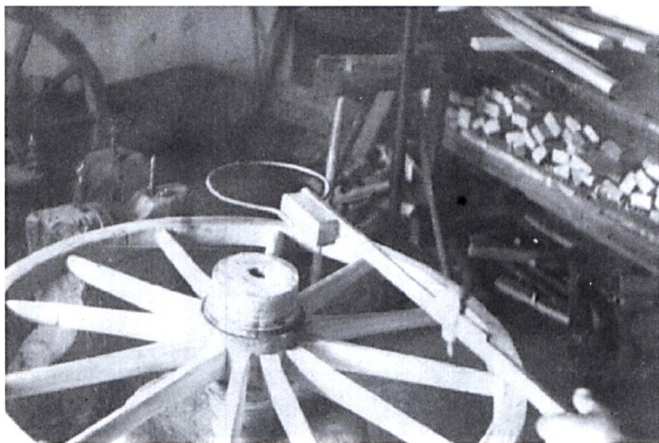
41. sz. kép: A kerék magasságának kijelölése
