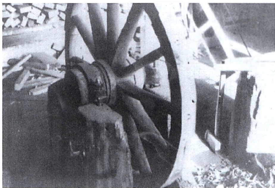
10. sz. kép: A kerékszék s benne egy rögzített kerék
