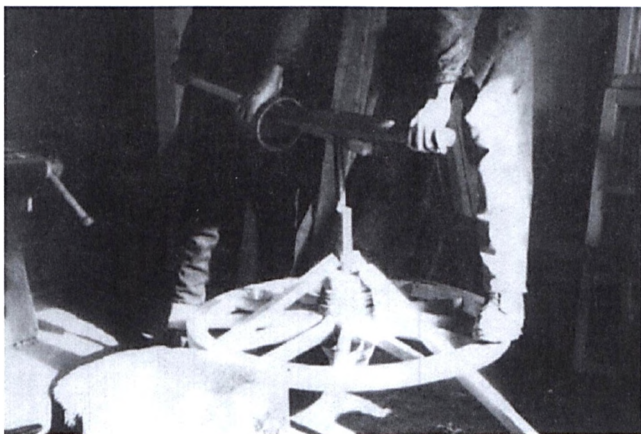
46. sz. kép: A kerékpuskázás
