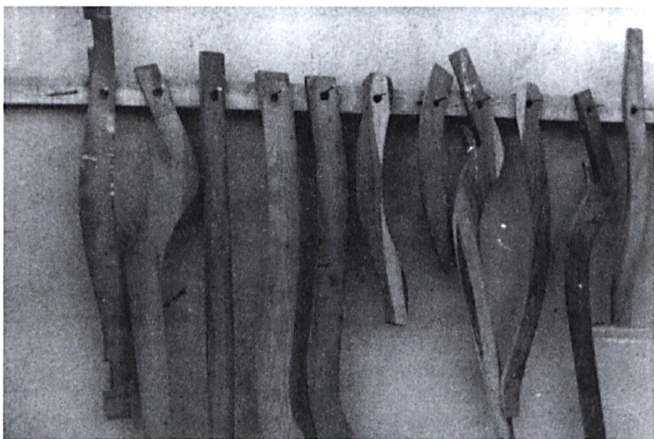
15. sz. kép: Minták vagy sablonok (lőcs, saráglya stb. mintája)
