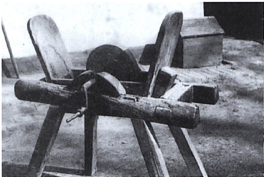
19. sz. kép: Kézi hajtású kösörűkő
