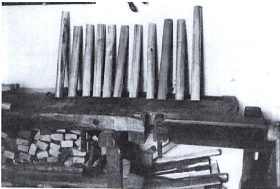
8. sz. kép: Gyalupad küllőkkel
