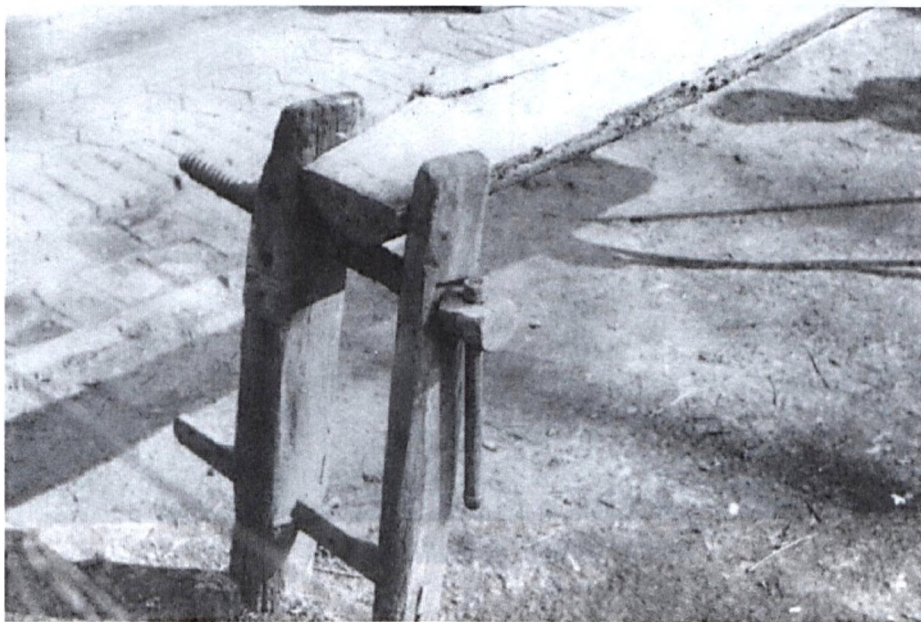
1. sz. kép: A satu
