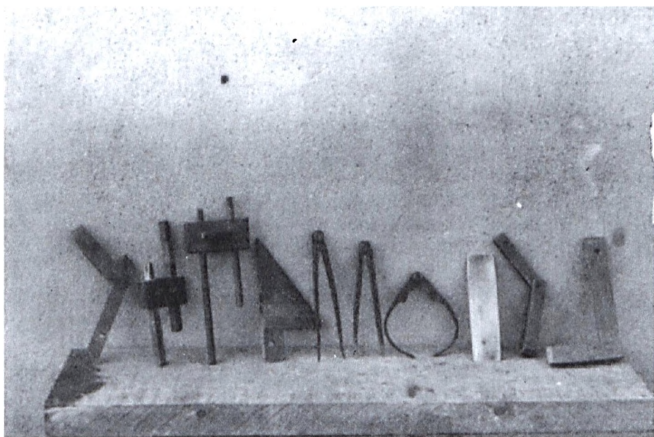
24. sz. kép: Bognárszerszámok (körzők, vinkli stb.)
