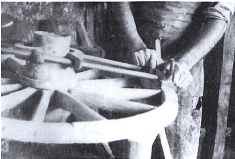
48. sz. kép: A keréktalp díszítése staubgyaluval
